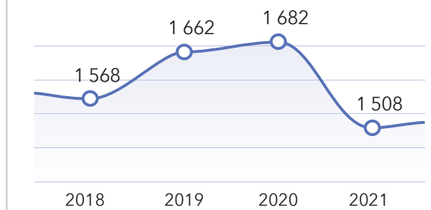
Рис. 7.4 Динаміка проведених заходів з вимірювання параметрів телекомунікаційних мереж у 2018-2021 роках Кількість заходів
