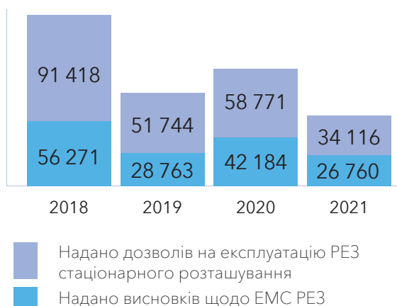
Рис. 7.7 Надання висновків щодо електромагнітної сумісності РЕЗ та дозволів на їх експлуатацію
